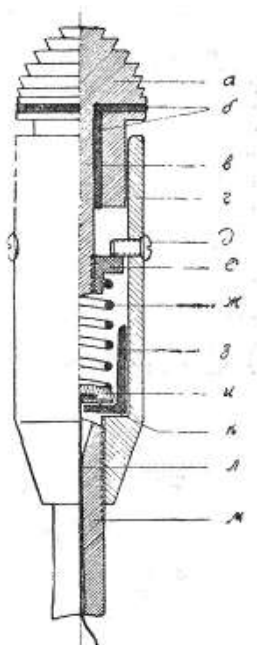
Рис. 55. Наконечник электрифицированной рапиры:
